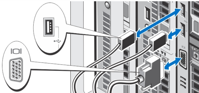
図 6. キーボード、マウス、およびモニタの接続
